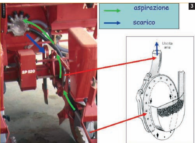
2 Particolare dell'apertura di scarico della ventola centrifuga di una seminatrice pneumatica da mais
